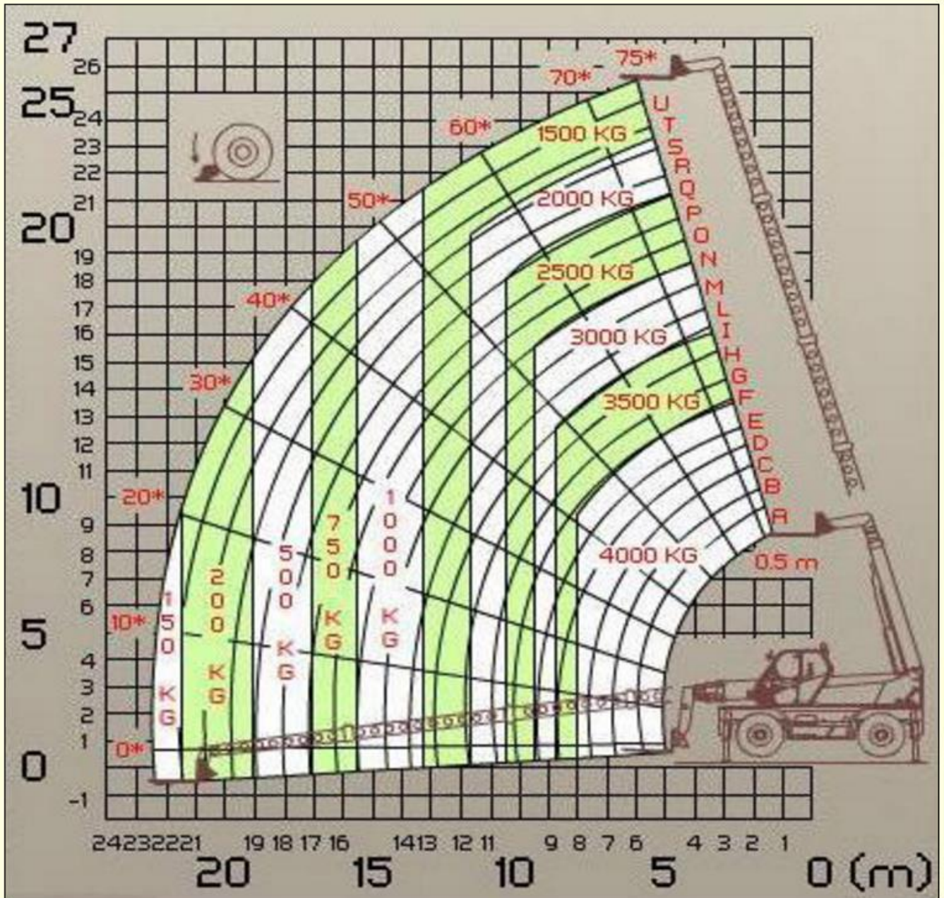
MERLO ROTO 40.30 MCSS – TABEL OP STEMPELS
